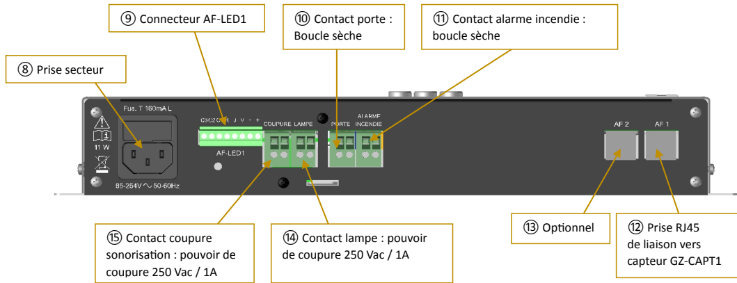
Figure 3. L'afficheur AF-VAL1 – Vue de face
